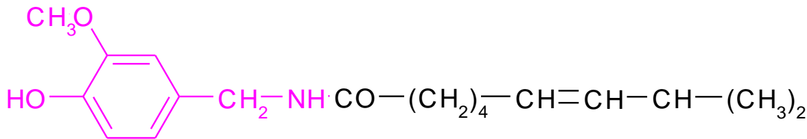
kapsaicin
