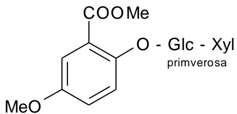
primulaverosid
