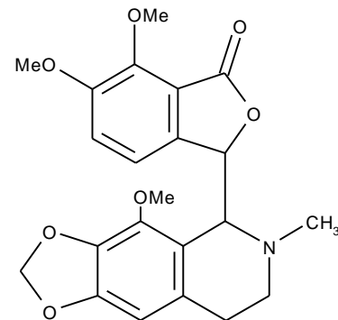
noskapin
