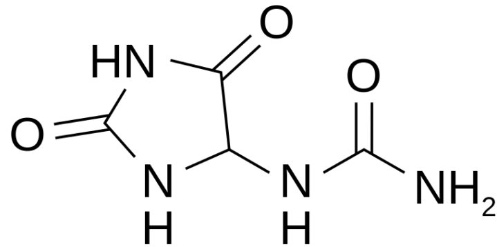
allantoin
