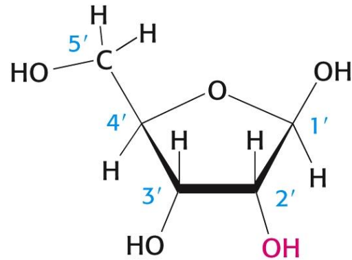
Ribose
