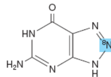
8-Azaguanine
