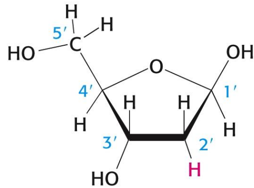
Deoxyribose
