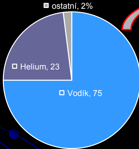
Složení vesmíru
