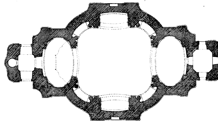
Obr. 17. Půdorys chrámu barokního.
