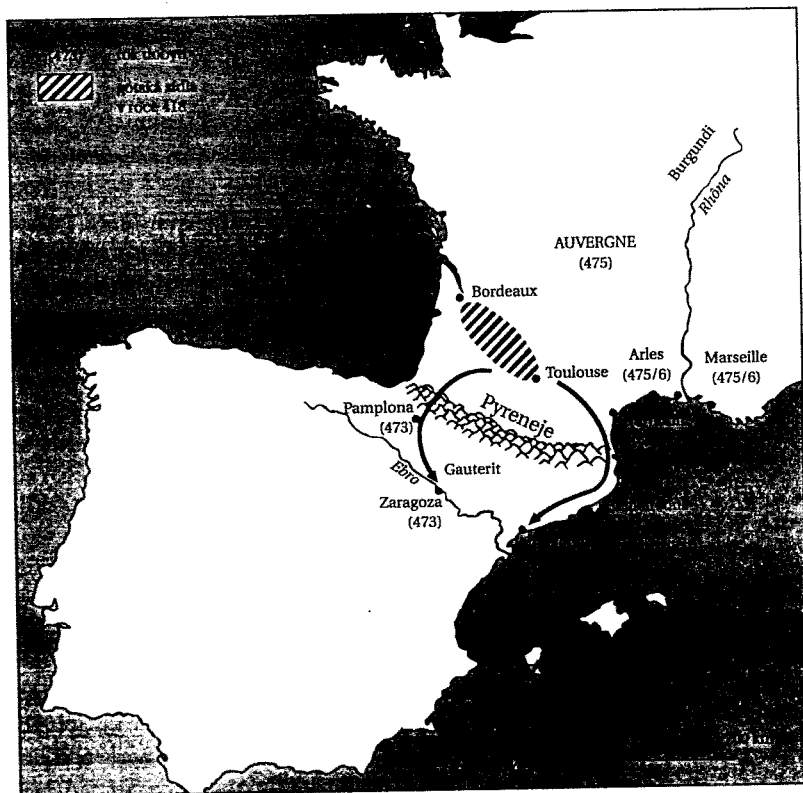
Eurichovy výboje
