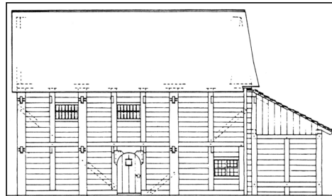
Ideální rekonstrukce měšťského domu s dřevěným sklepem a s hrázděním (podle Davida Mertly)
