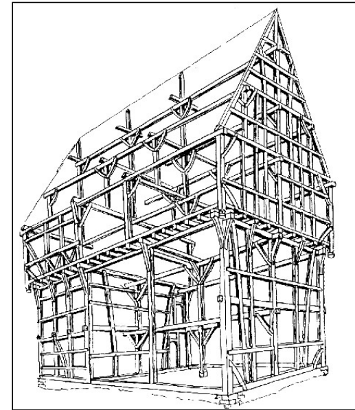
Rekonstrukce kostry hrázděného měšťského domu z 15. století (Pfistermeister 1993)
