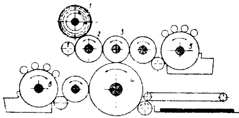
Schéma uspořádání válců u první Bullockovy rotačky
