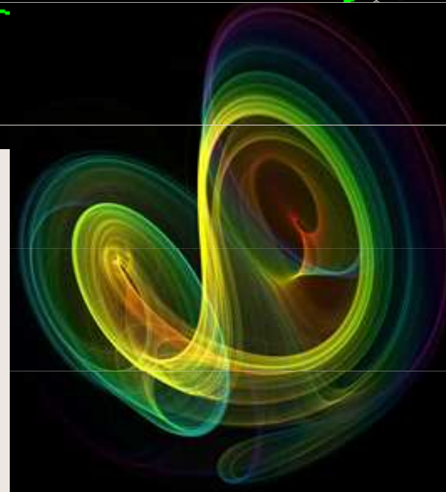
Lorenzův atraktor
