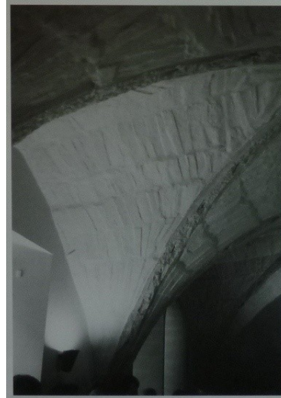
Otisky bednění, připraveného z úseků krátkých prken (možná šindelů), na kápičích křížových klenb z 14. století – na fotografii z budovy pražského Karolina na Starém Městě, na kresbě z křížové chodby augustiniánského kláštera v Roudnici (J. Pešta).
