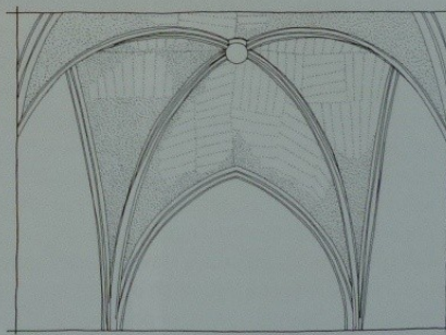
Otisky bednění, připraveného z úseků krátkých prken (možná šindelů), na kápičích křížových klenb z 14. století – na fotografii z budovy pražského Karolina na Starém Městě, na kresbě z křížové chodby augustiniánského kláštera v Roudnici (J. Pešta).
