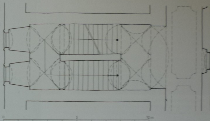
Základní typ renesančního zámeckého schodiště – dvouramenné s plnou vřetenovou zdí, nad podestami s plochými klenbami křížového typu. Komorní Hrádek u Benešova, 1616 (M. Rykl).
