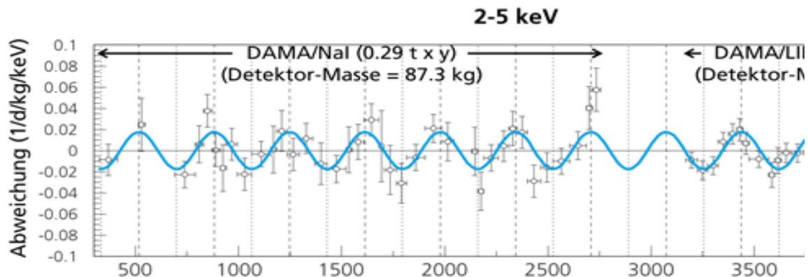
Abb. 1: Zeitliche Variation der registrierten Zusammenstöße in den Detektoren des DAMA-Experiments (aus Bernabei 2008a). Aufgetragen ist die Abweichung vom zeitlichen Mittelwert für den Energiebereich 2-5 keV* als Funktion der Zeit. Als Nullpunkt der Zeitachse wurde der 1. Januar des ersten Jahres der Datennahme gewählt. Die durchgezogene Linie zeigt eine Oszillation mit einer Periode von einem Jahr und einem Maximum jeweils am 2. Juni des Jahres.
