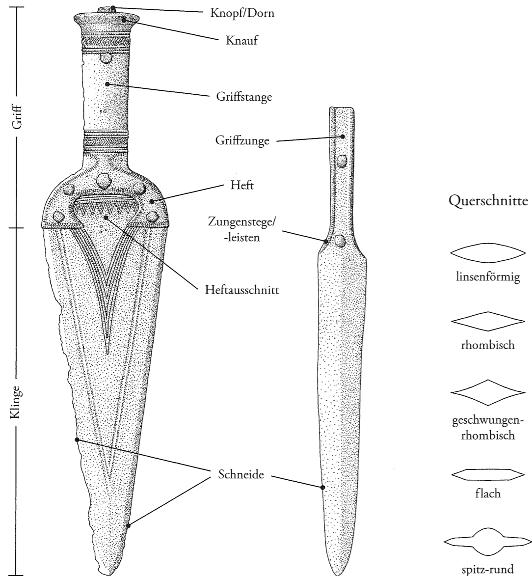
Abb. 1. Terminologie der Dolchelemente sowie deren charakteristische Klingenschnitte
