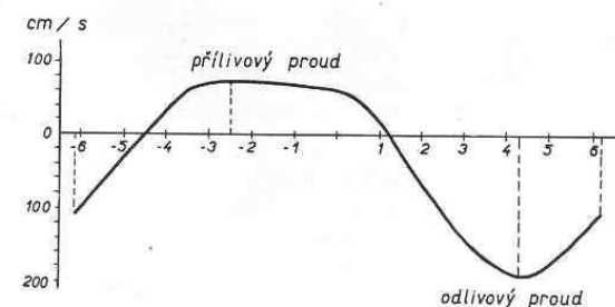
Obr. 7.33. Křivky udávající rychlosti výčasových proudů. Na vodorovné ose je zachycen čas v hodinách. Obě křivky jsou výsledkem měření v době skočného přílivu. Nahoře u Wilhelmshavenu, dole u Cuxhavenu. U spodní křivky lze zřetelně pozorovat větší maximální rychlosti odlivového proudu než proudu přílivového. Podle G. Sagera (1959).
