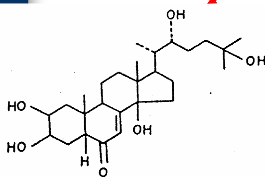
Ecdysone
