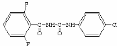
diflubenauron
