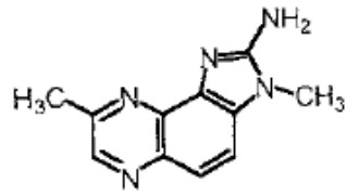
MeIQx
