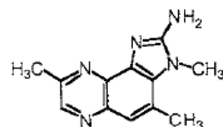
DiMeIQx
