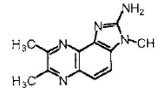
7,8-DiMeIQx
