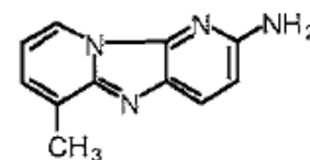
Glu-P-1
