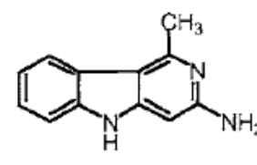
Trp-P-2
