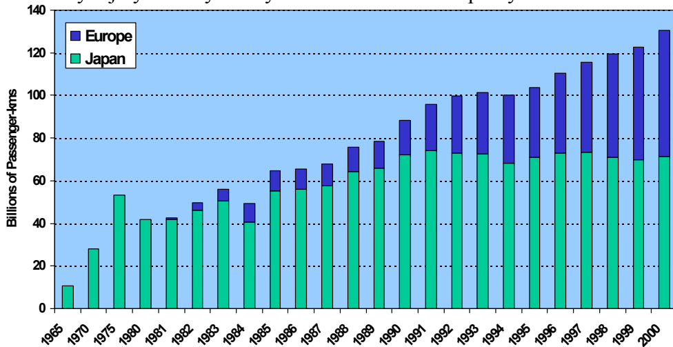
Obr. 20: Vývoj výkonů vysokorychlostní železniční dopravy
