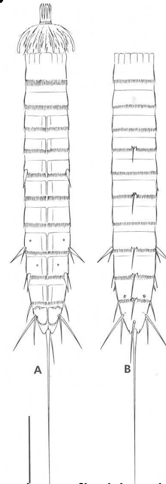
Zelinkaderes floridensis (Cyclorhagida), samice: A - introvert vychlípán, břišní strana; B - introvert zatažen, uzavřen 2. zonitem, hřbetní strana; měřítko 100 \mu m
