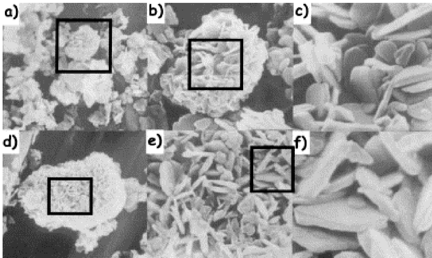
STEM neozářené (a, b, c) a laserem ozářené (d, e, f) olovnaté běloby ( 2\text{PbCO}_3 \cdot \text{Pb(OH)}_2 ) zvětšení \times 5 (a, d), \times 15 (b, e) a \times 50 (c, f) tis. Oba povrchy jsou velmi podobné, bez zjevných rozdílů.
