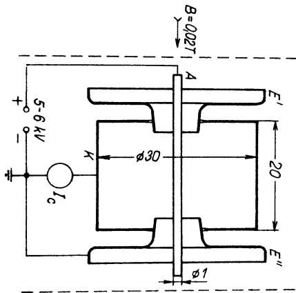
Výbojový manometr - inverzní magnetron
