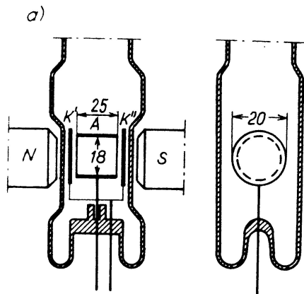
Výbojový manometr - Penning
