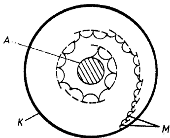
Obr. 7-30. Dráhy elektronu v inverzním výbojovém manometru
