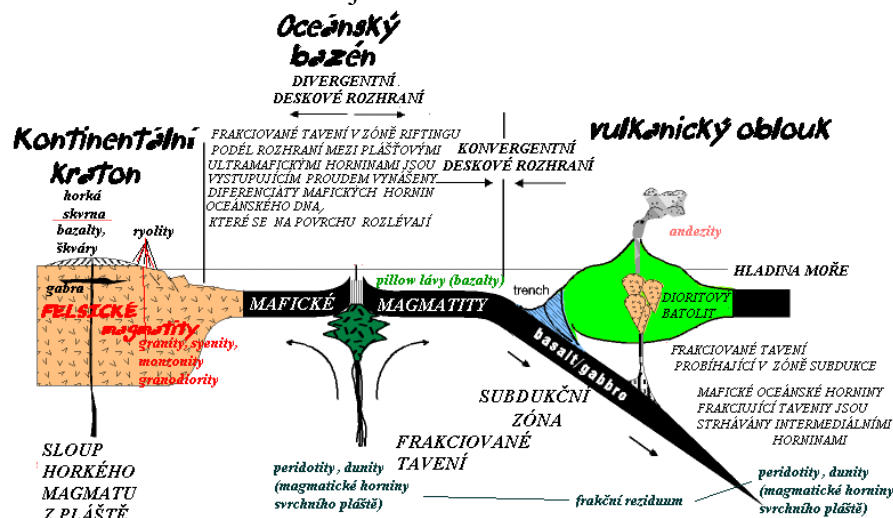
Obr. 26 Tvorba litosféry – frakcionace litosférických desek
