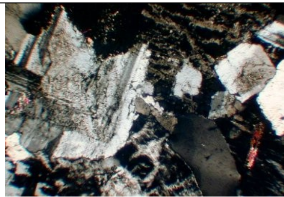
holokrystalický granit
