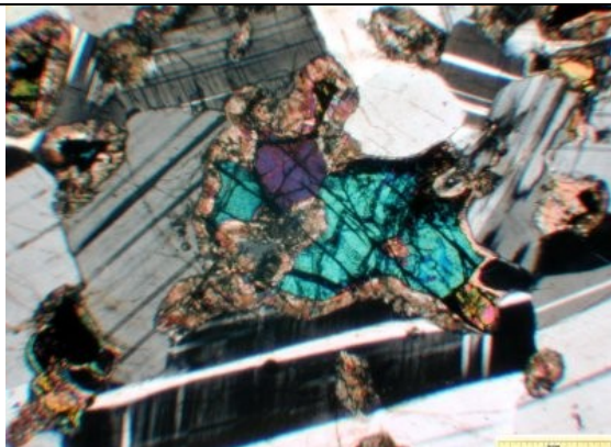
granuloofitická
