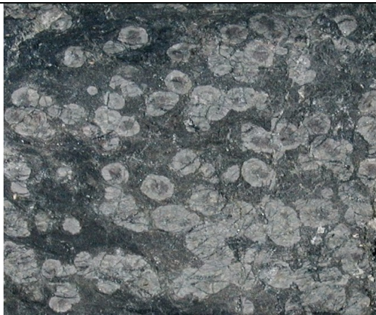
Sférolitická – ve struktuře jsou přítomny sférolitické útvary minerálů (makroskopicky nápadné okrouhlé útvary) – neplést si s amygdaloidní)
