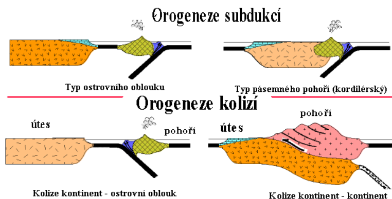
Obr. 27 Typy orogenezi
