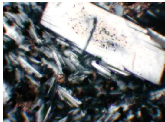
hemikrystalický andezit
