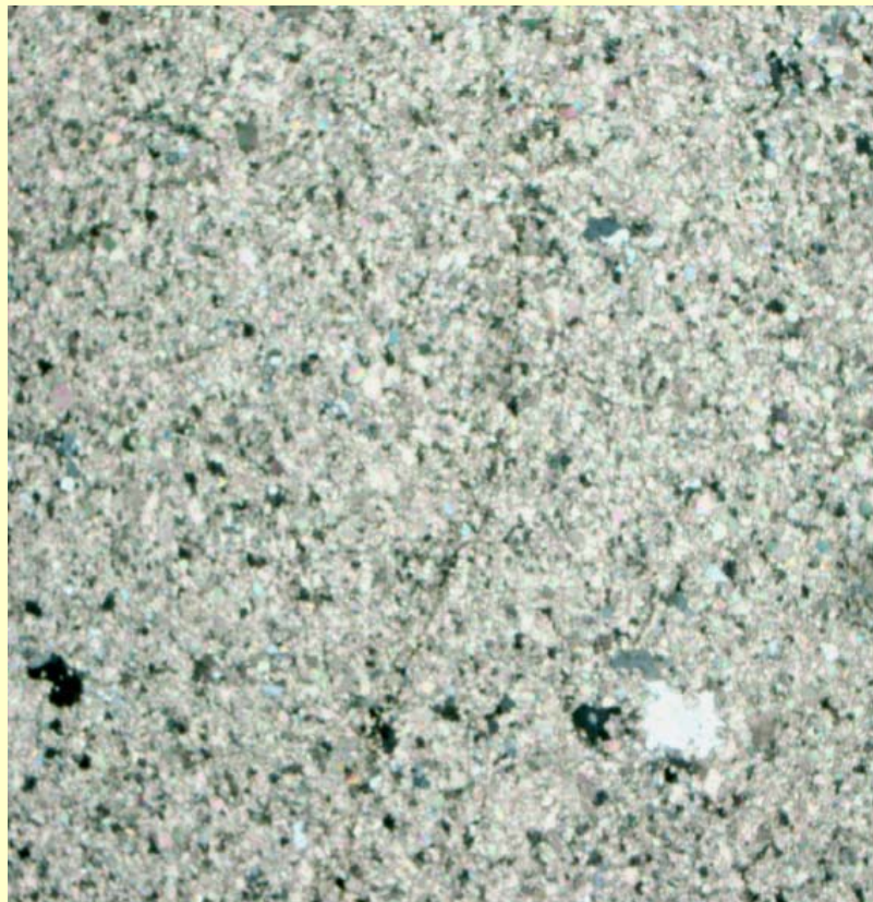
Kalcitická břidlice s křemenem (Mongolsko)
