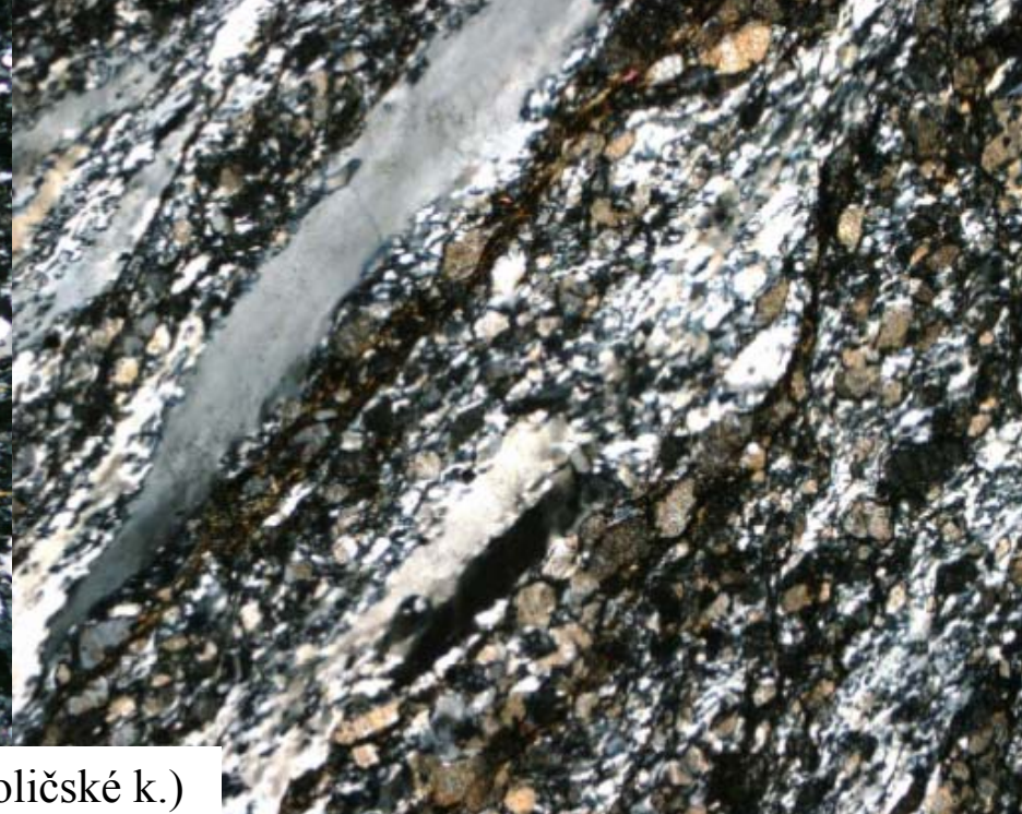
Kataklazit (poličské k.)
