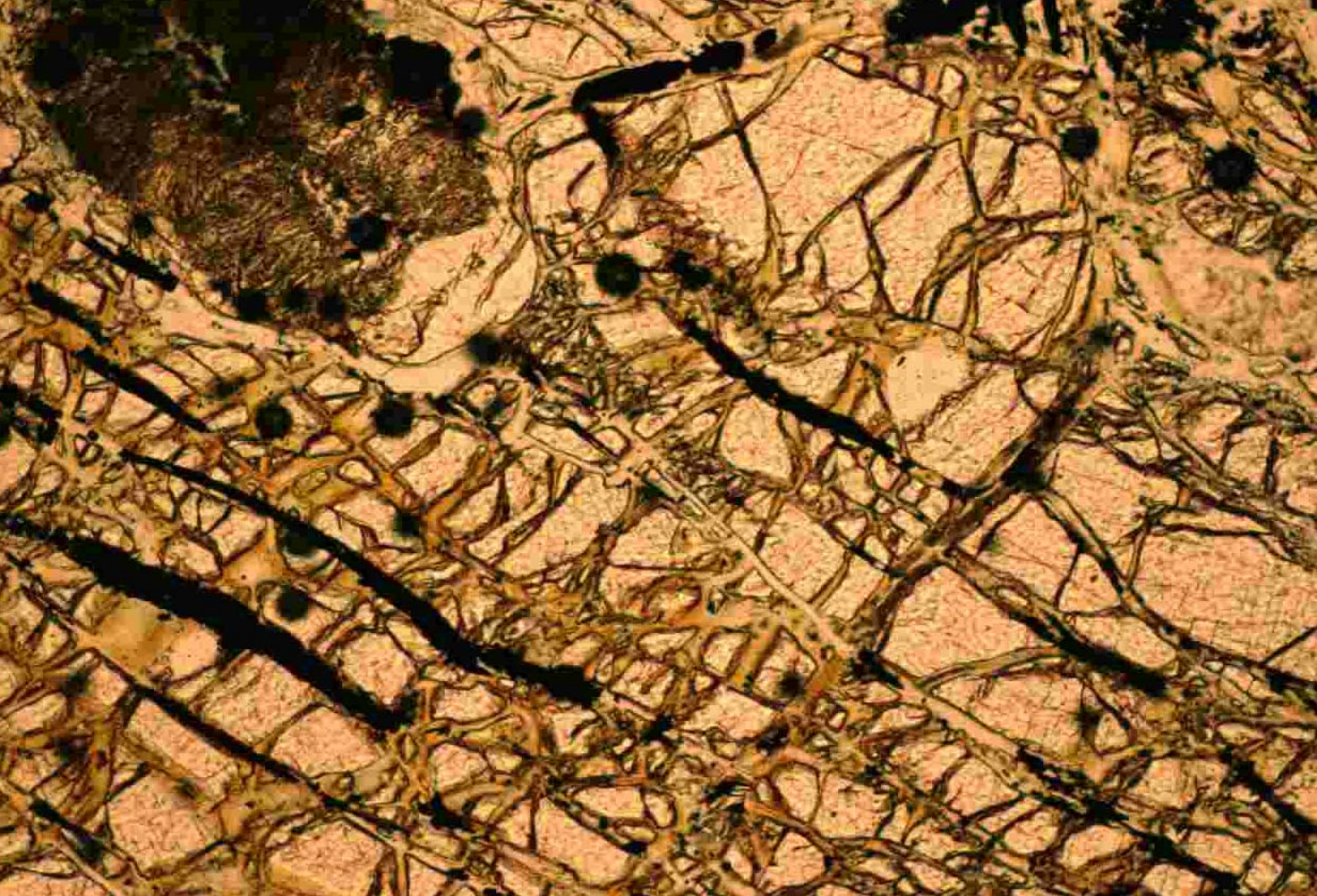
Metaperidotit (Horní Bory)
