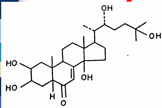
Ecdysone
