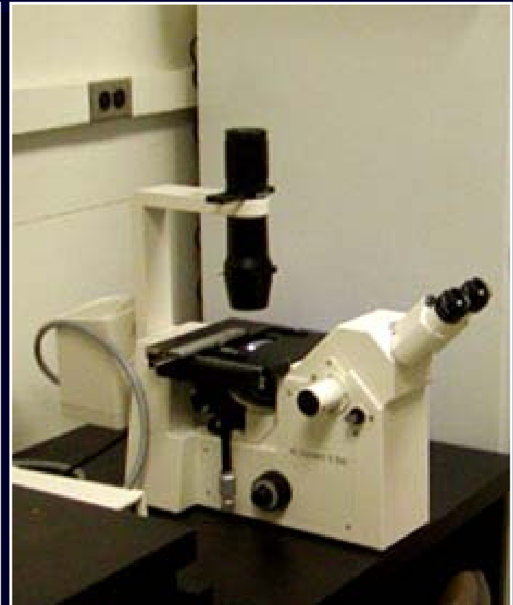
invertovaný mikroskop
