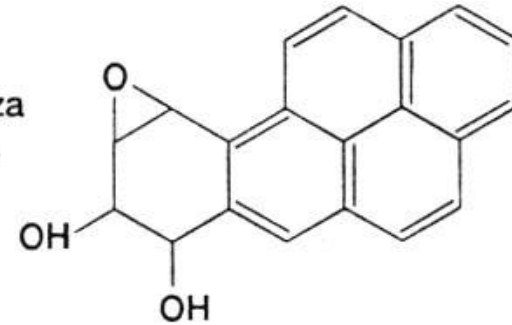
9,10-epoxy-benzo[a]pyren-7,8-diol
