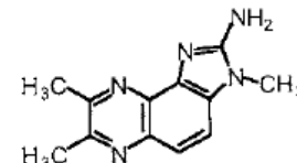
7,8-DiMeIQx
