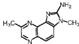
MeIQx
