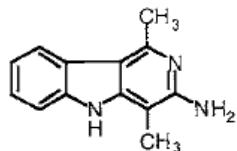
Trp-P-1
