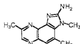
DiMeIQx
