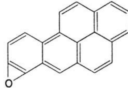
7,8-epoxy-benzo[a]pyren
