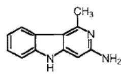
Trp-P-2
