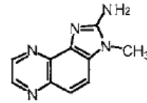
IQx
