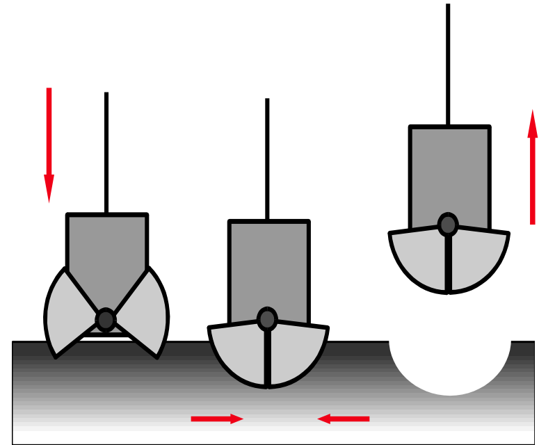
Grab probe
