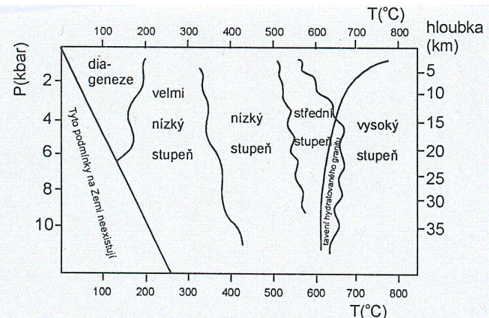
Obr. 1-1. Schematický PT (tlak, teplota) diagram s vyznačením polí pro stupně metamorfózy a diagenezi. V diagramu je také vyznačena křivka tavení hydratovaného granitu a pole podmínek, které na Zemi neexistují.
