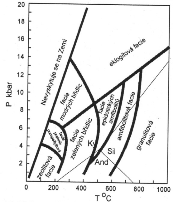
Obr. 5-5. P-T diagram s hlavními metamorními facie a trojným bodem Al_2SiO_5 , podle Holdawaye 1971. Převzato ze Speara (1993).
