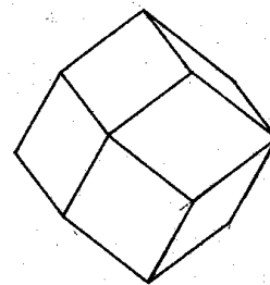
dvanáctistěn kosočtverečný
