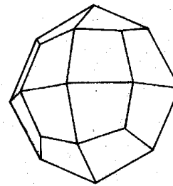
čtyřiadvacetistěn deltoidový
