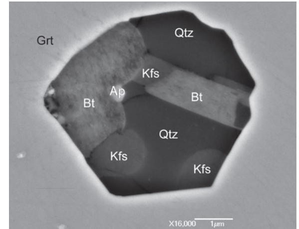
Inkluze granitu v granátu Sawyer 2011
