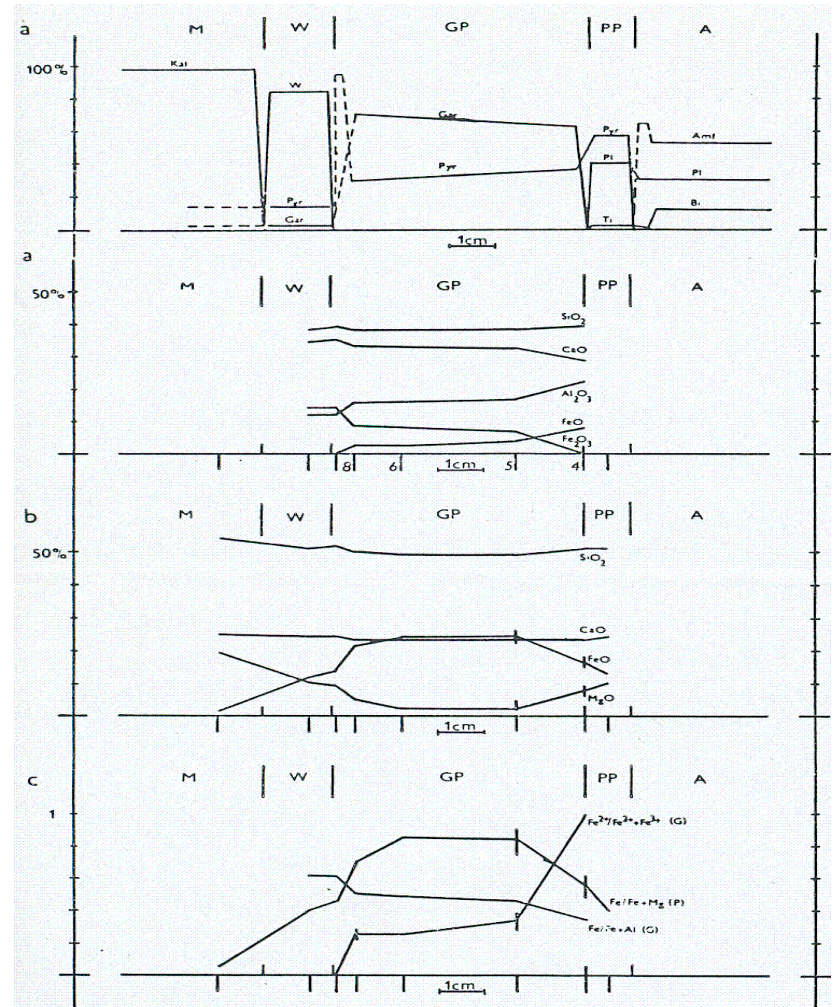
Obr. 2. Chemické složení granátů a pyroxenů přes skarnové zóny. Fig. 2. Chemical composition of garnets and pyroxenes across skarn zones. Svislími čarami jsou označena místa analýz na mikrosondě. Spot locations of microprobe analyses are marked by perpendicular lines. Diskuse v textu. — Discussion in text.
