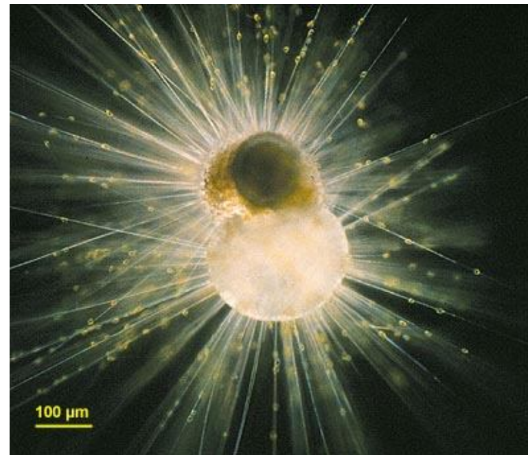
G. bulloides
