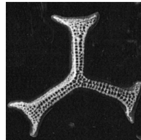
Halesieum tricanthum
