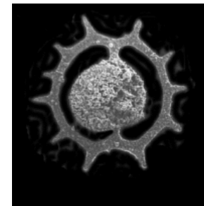
Acanthoicircus tympanum
