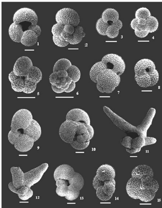
Globigerina
