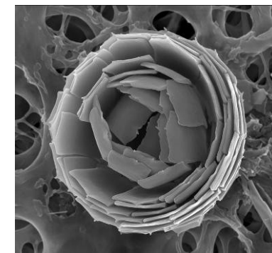
Florisphaera profunda
