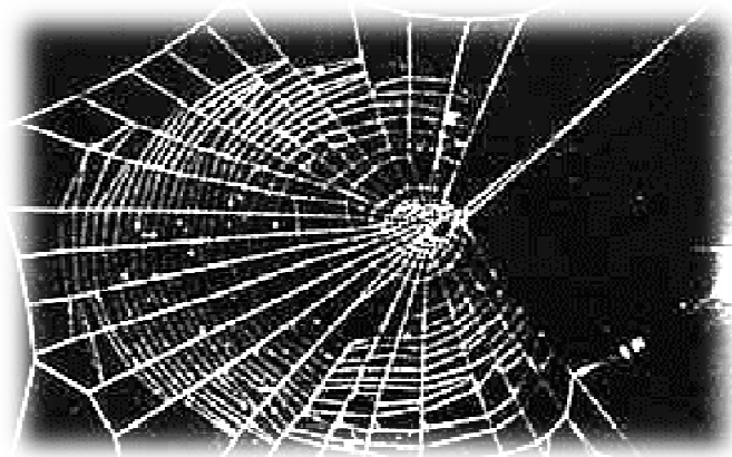
meskalin
