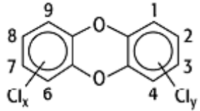
Polychlorodibenzo-p-dioxine (PCDD)
