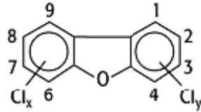
Polychlorodibenzofurane (PCDF)
