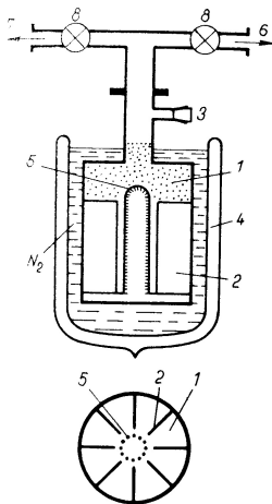
Obr. 4.108. Zeolitová vývěva
