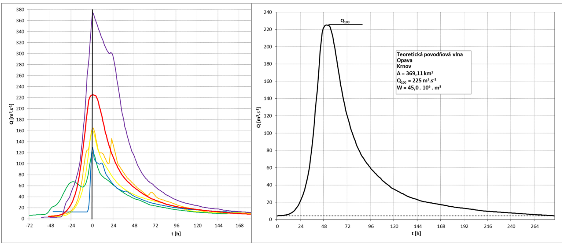
Schematizace hydrogramů
