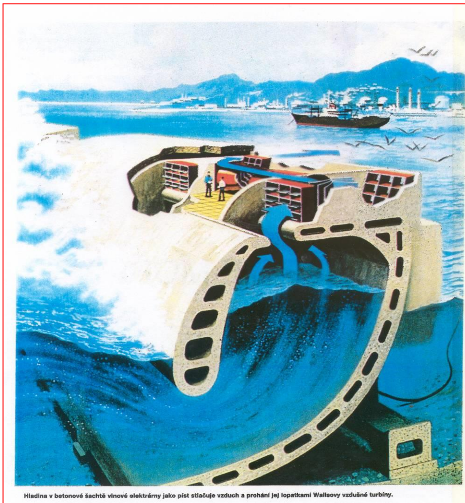
Hladina v betonové šachtě vinové elektrárny jako píst stlačuje vzduch a prohání jej lopatkami Walleovy vzdušné turbíny.
