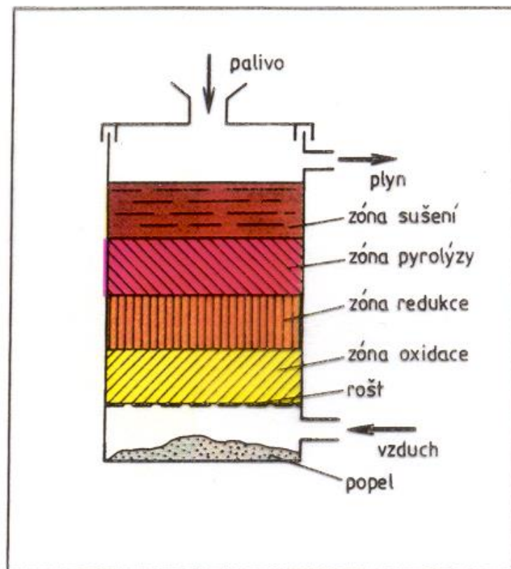
Protiproudý zplyňovač
