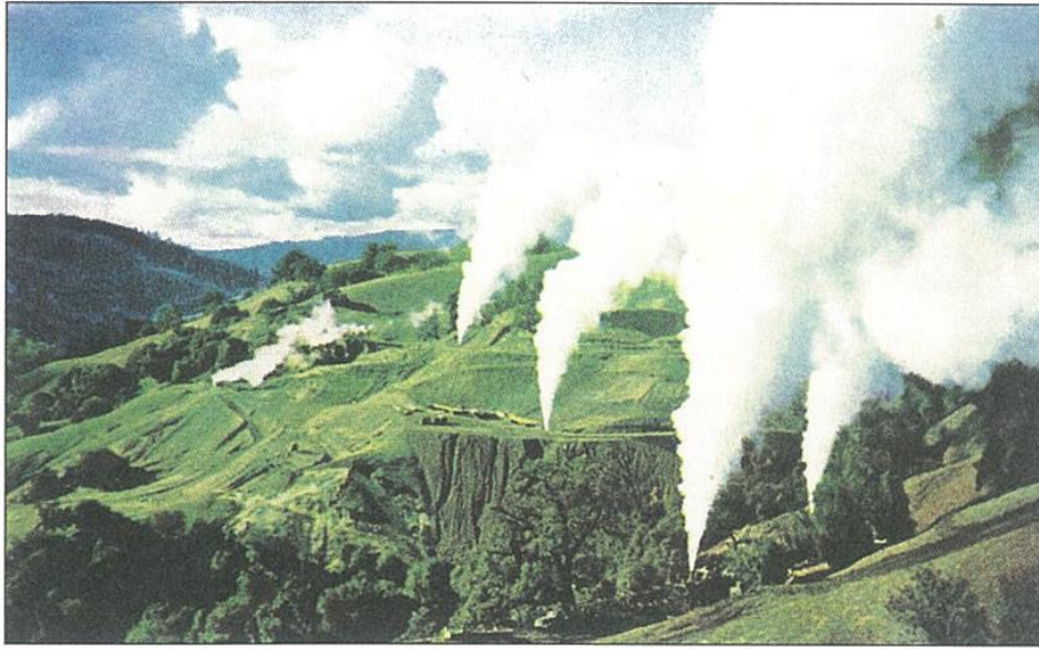
Geotermální pole The Geysers v Kalifornii.
