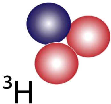
tritium
