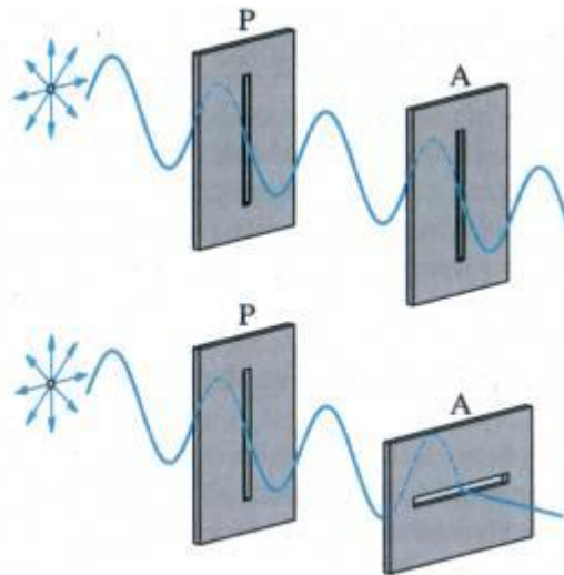
Model polarizátoru a analyzátoru
