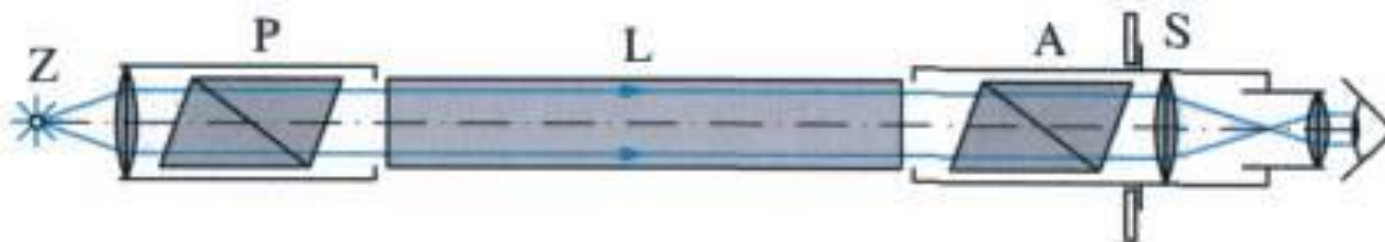
Princip polarimetru
