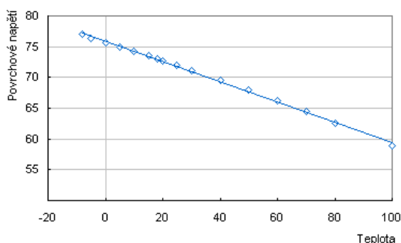
Obr. 6. Závislost povrchového napětí na teplotě.
