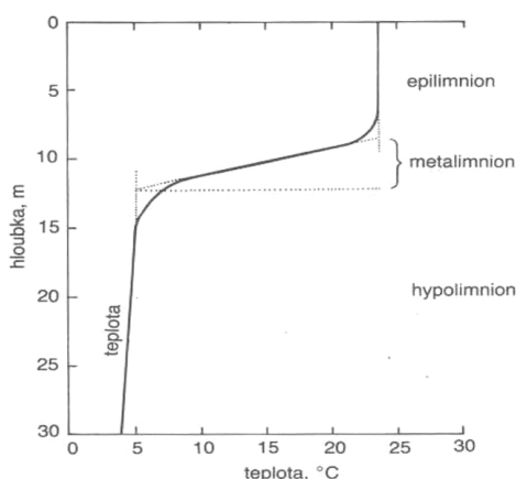
Obr. 4. Letní teplotně hustotní stratifikace ve stojaté vodě (idealizovaný model)
