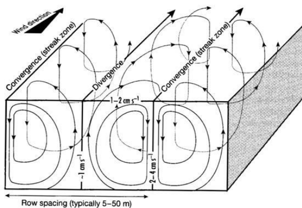
Obr. 12 Langmuírovy spirály – velikost a rychlost proudění.
