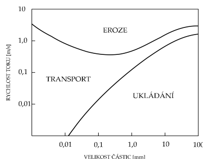
Obr. 16 Vztah rychlost proudění a velikosti unášených částic ve vodním sloupci.
