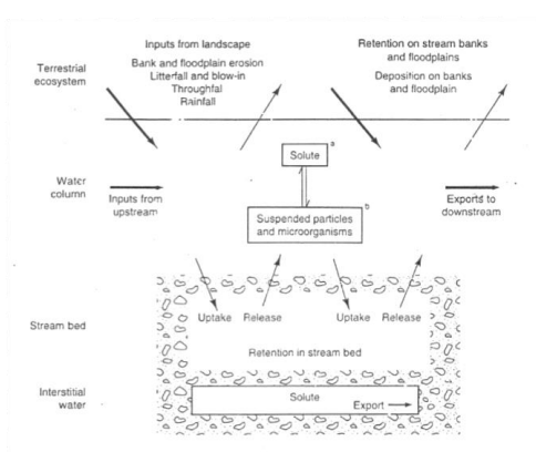
Obr.38 Vstupy a výstupy organické hmoty v obecném vodním tělese
