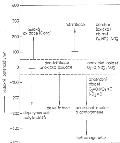
Obr. 22. Typy vodního prostředí dle kyslíkového režimu (oxidace – redukce).
