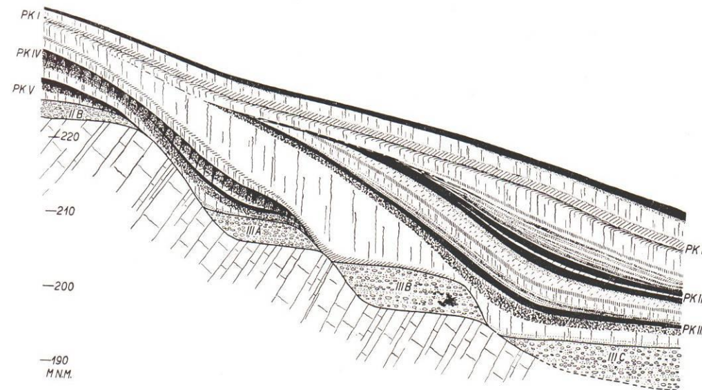
33. Náčrt úložných poměrů sprašové série na souboru stupňů říčních teras (podle poměrů v údolí Vltavy pod Prahou). V podloží zvrásněné algonkium, terasy podle Q. Záruby (1943): II b — letenská, III a — dejvická, III b — Karlova náměstí, III c — veltruská (členy sprašové série značeny stejně jako na obr. 17 a 30). (Ložek 1973)
