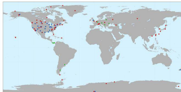
Obr. 5. Geografická distribuce stanic měřících intenzitu UV záření a přispívajících do WUOUC rozdělených podle typu používaného přístroje s využitím dat WUOUC (2013) a ESRI World v souřadném systému WGS 1984
