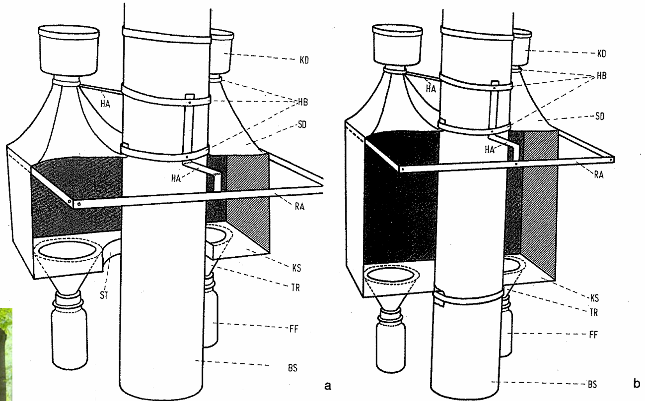
Otev ený stromový fotoeklektor Uzav ený stromový fotoeklektor (Výrobek firmy Behre; z Mühlenberg, 1989)
