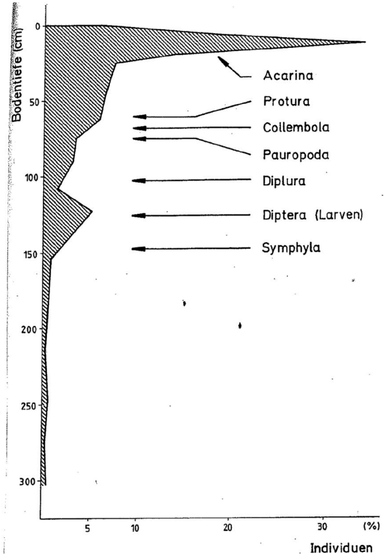
Abb. 66: Vertikalverteilung der Arthropoden in landwirtschaftlich genutzten Bŕden, und durchschnittliche Besiedlungstiefe der Tiergruppen (Daten nach PRICE und BENHAM 1977).
