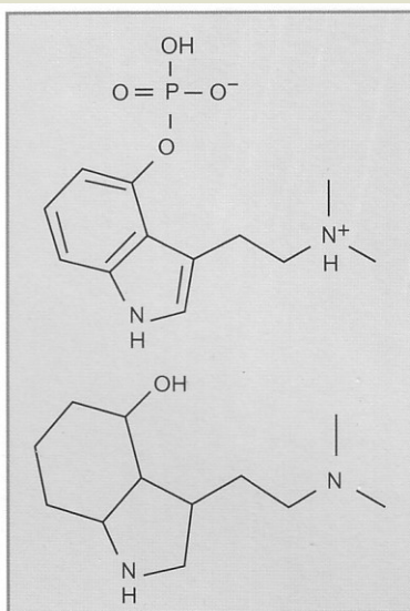
Obr. 30. Strukturní vzorce psilocybinu (nahoře) a psilocinu (dole)
