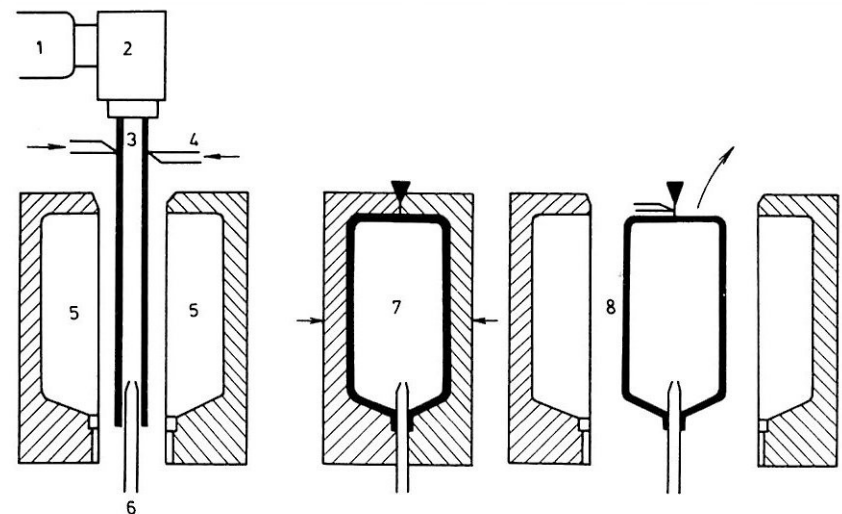
Obr. 24.3. Vytlačování s vyfouknutím pro výrobu dutých těles (vyfukování spodem pomocí trnu)
