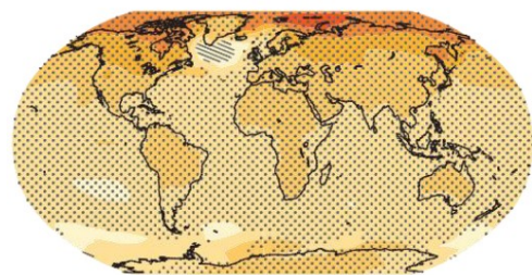
RCP 2.6
