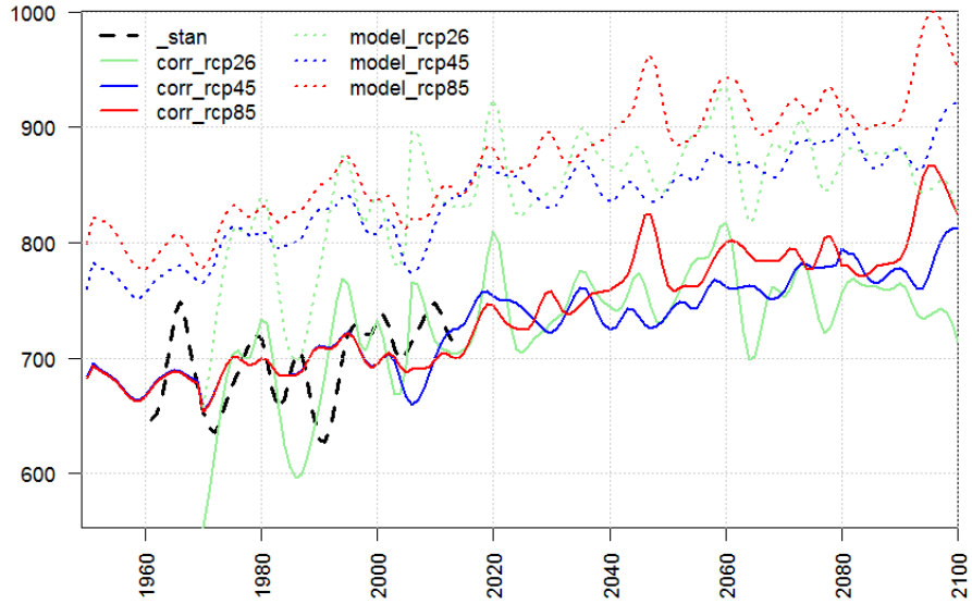
monthly-sra N_YEAR
