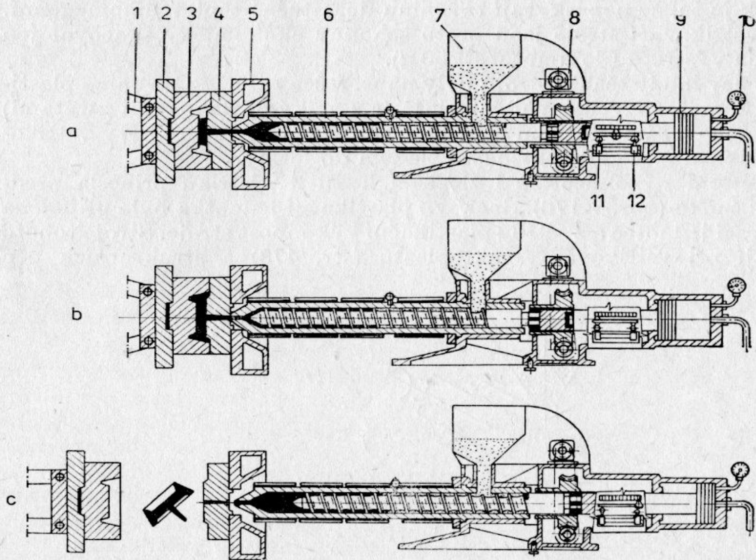
Obr. 7-177. Pracovní cyklus vstřikovacího stroje se šnekovou plastikační jednotkou a) vstřikování, b) dotlačování, c) vyjmutí výstřiku z formy; 1 — uzavírací mechanismus, 2 — pohyblivá upínací deska, 3 — tvárnice, 4 — tvárník, 5 — nepohyblivá upínací deska s otvorem pro trysku, 6 — vstřikovací válec, 7 — násypka, 8 — hydraulický motor pro pohon šneku, 9 — hydraulický válec, 10 — tlakoměr, 11 — koncový spínač dotlačování, 12 — koncový spínač zpětného posunu šneku
