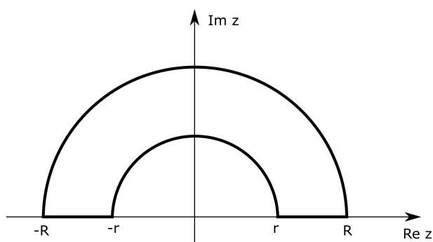
Obrázek 1: Křivka \mathcal{C} .
