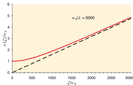
Obr. 5 Pološířka gaussovského svazku v závislosti na vzdálenosti šíření a asymptota k pološířce v nekonečno. Veličiny jsou vztaheny k pološířce svazku w_0 v počátku (nejušší místo svazku: sedlo či pas svazku), struktura platí pro jednu velikost w_0 vztahenou na vlnovou délku. Graf je ve svislém směru silně roztažený.
