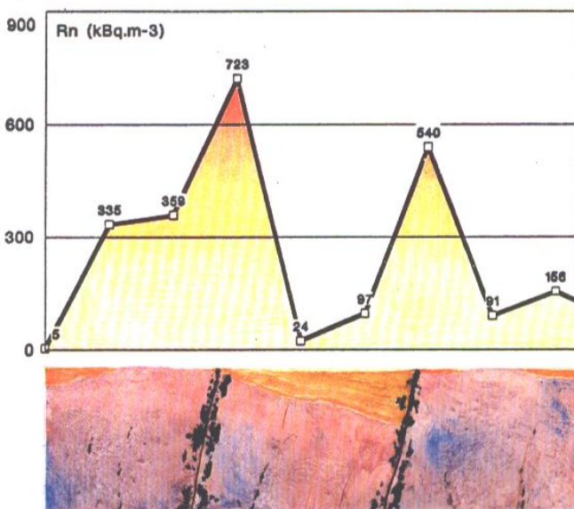
Uranové zrudnění na tektonické poruše se projevuje zvýšenou hodnotou objemové aktivity radonu (lokalita Kovářov u Milevska).
