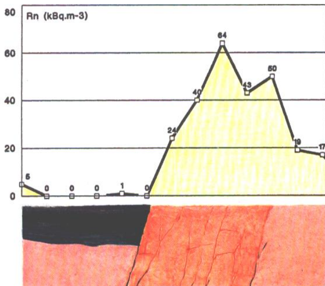
Vliv nepropustného jřlovitého pokryvu na snížení hodnoty objemové aktivity radonu. Pod jřlovou vrstvou vzniká bariérový efekt, radon migruje podél tektonické poruchy (lokalita Radvanov u Milevska).
