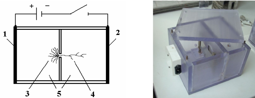
Obrázek 1: Vlevo foto výbojové komory, vpravo schéma diafragmového („bezelektrodového“) výboje: 1 – anoda, 2 – katoda, 3 – negativní plazmové kanály, 4 – pozitivní plazmové kanály, 5 – vodivý kapalný roztok.
