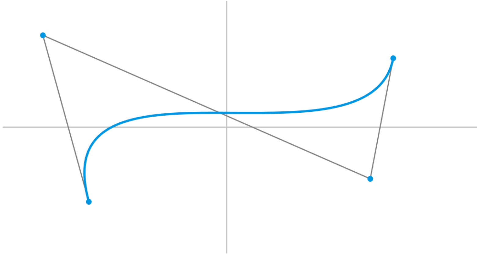
Obr. 1: Znáznění Bézierovy křivky
