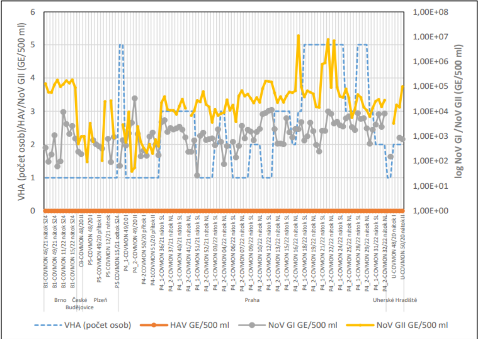
Obr. 6 Výskyt specifických oblastí genu virů HAV, NoV GI a NoV GII v odpadních vodách (2020-2022).
